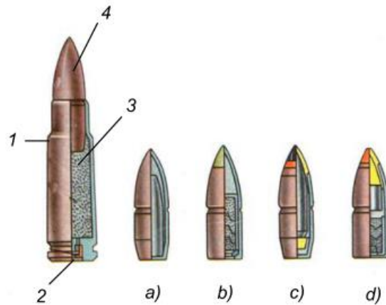
Hình 4-17. Đạn K56
