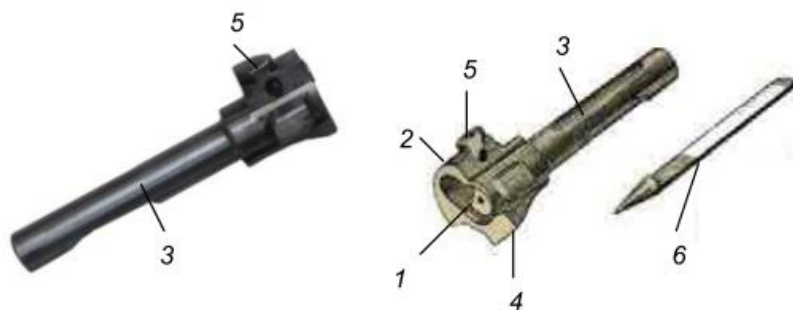
Hình 4-9. Khoá nòng
