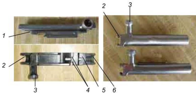
Hình 4-36. Bệ khoá nòng 1. Rãnh lượn ; 2. Khe lắp kẹp đạn ; 3. Tay kéo bệ khoá nòng ; 4. Mấu mở khoá ; 5. Mấu đóng khoá ; 6. Lỗ chứa bộ phận đẩy về.
