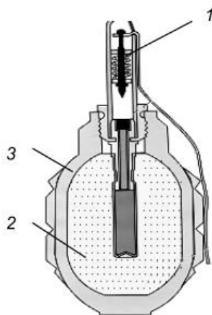
Hình 6-2. Cấu tạo lựu đạn \Phi 1 1. Bộ phận gây nổ ; 2. Thuốc nổ ; 3. Vỏ lựu đạn.
