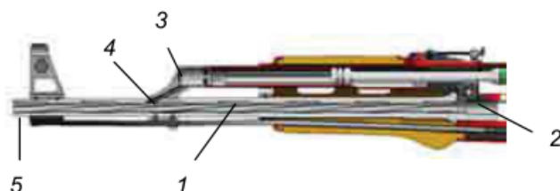
Hình 4-3. Nòng súng
