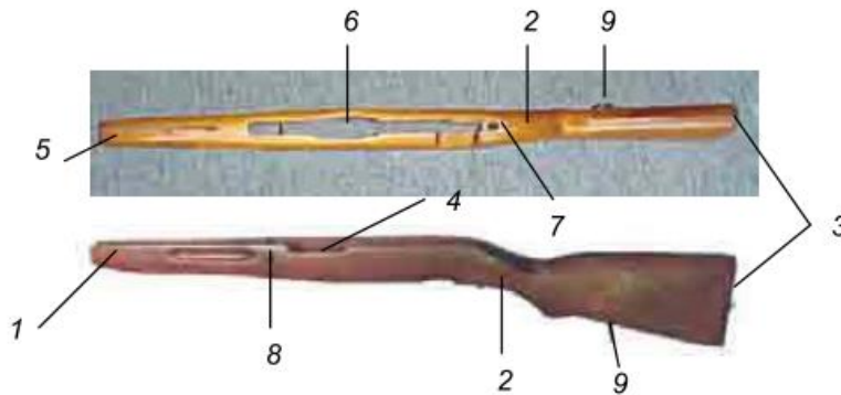
Hình 4-42. Báng súng
