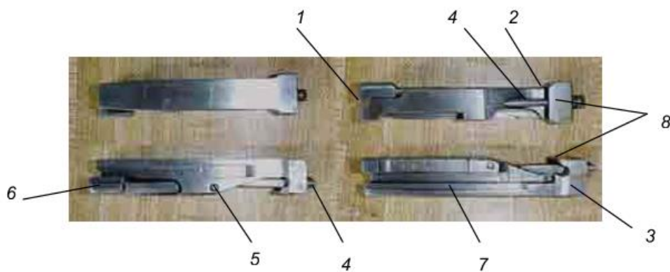
Hình 4-37. Khoá nòng
