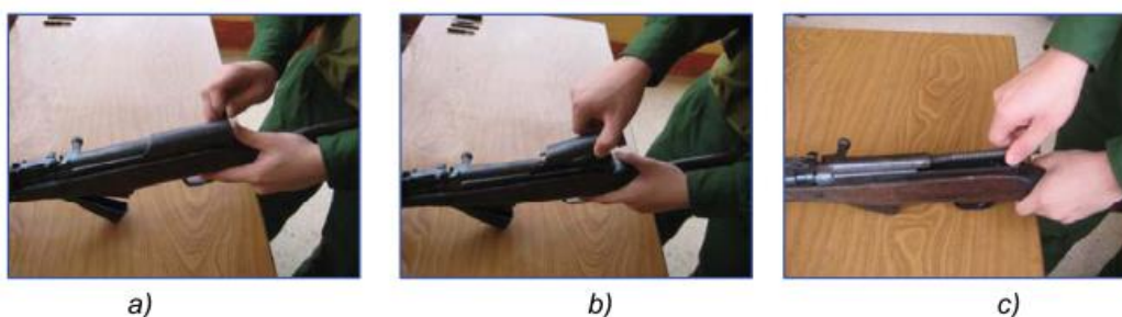
Hình 4-49. Tháo nắp hộp khoá nòng a, b) Tháo nắp hộp khoá nòng ; c) Tháo bộ phận đẩy về.
