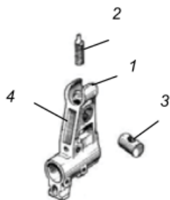
Hình 4-4. Đầu ngắm
