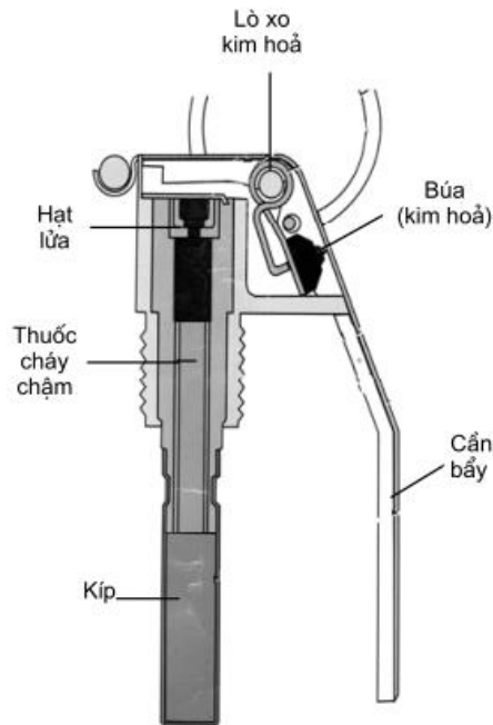
Hình 6-5. Cấu tạo bộ phận gây nổ
