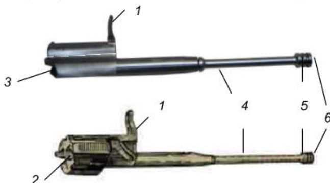
Hình 4-8. Bệ khoá nòng và thoi đẩy
