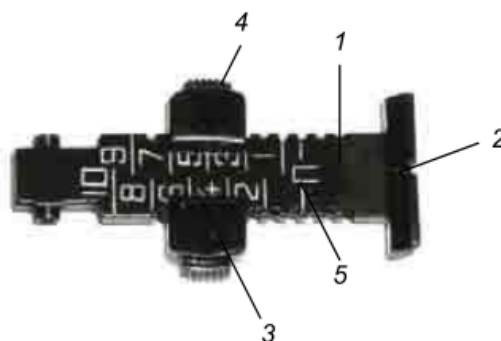
Hình 4-33. Thước ngắm
