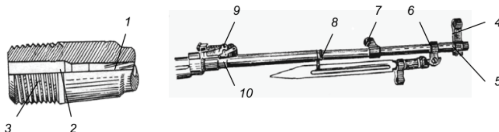
Hình 4-31. Nòng súng
