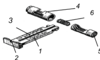
Hình 4-5. Thước ngắm
